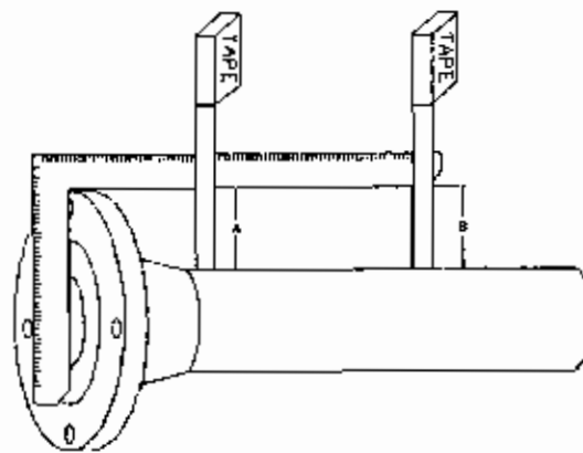
A-B=TOLERANCE
