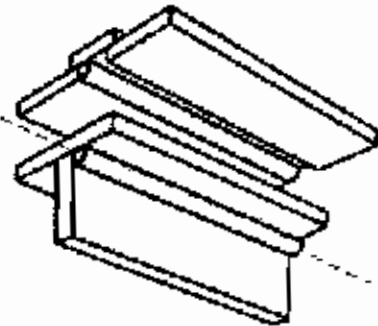
(D) OVERHEAD WELDING TEST POSITION 4F
