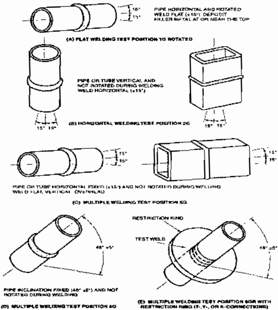
شکل ۲-۹: حالات جوش شیباری (لب به لب) بر اساس نحوه قرار گرفتن لوله (1G ~ 6G)
