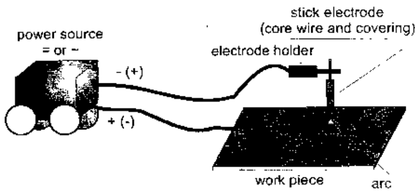
شکل ۲-۱۴: تجهیزات مورد نیاز در روش SMAW
