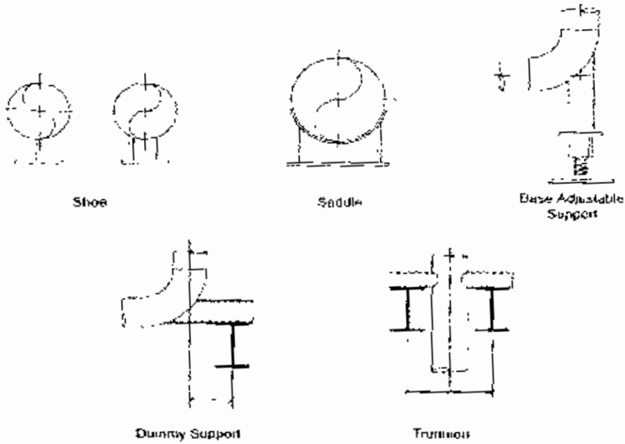
شکل ۲-۴: ساپورت‌های ساده Simple
